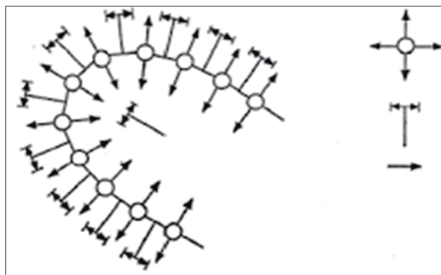
Figura 2. Diagrama de representação de indivíduos interdependentes (família, estado, grupos etc.)
